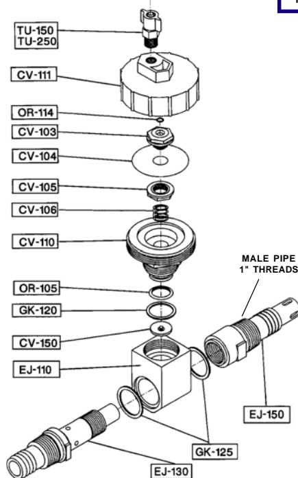
Ejector
